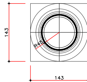
2 PLANTA DO PEDESTAL Esc. 1/25
