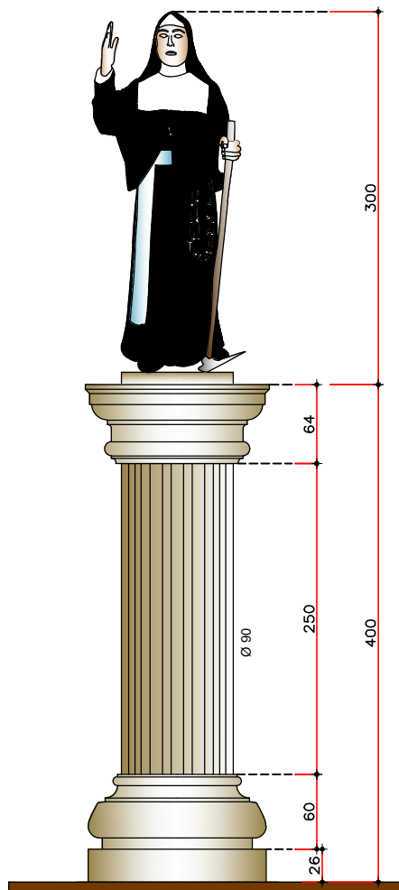
1 ELEVAÇÃO FRONTAL Esc. 1/25
