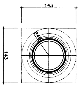
2 PLANTA DO PEDESTAL Escala: 1/25
