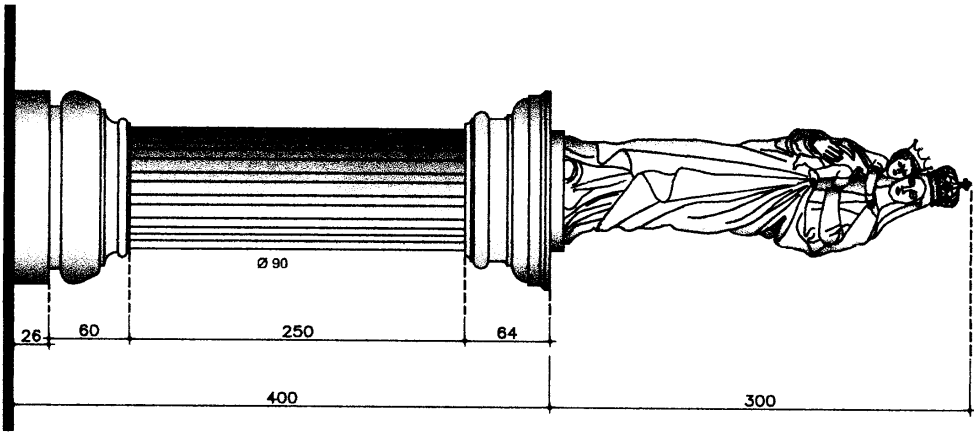
1 ELEVACÃO FRONTAL Esc. 1/25
