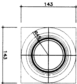
2 PLANTA DO PEDESTAL Esc. 1/25
