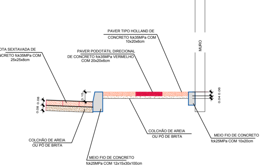
Seção Tipo Calçadas - Esc. 1/25
