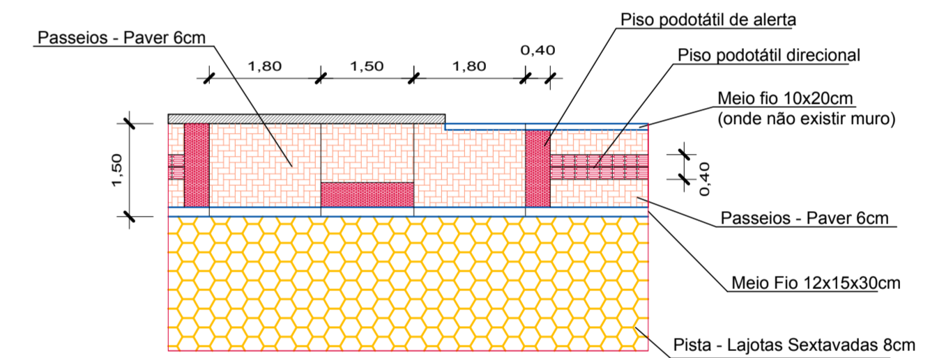
Detalhe do Rebaixamento das Calçadas e Faixas de Pedestres - Esc. 1/75
