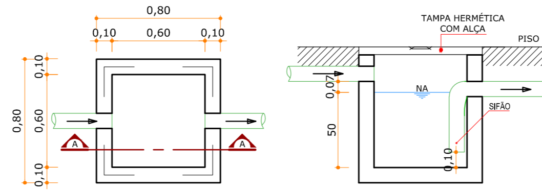
PLANTA ESCALA | 1:25
