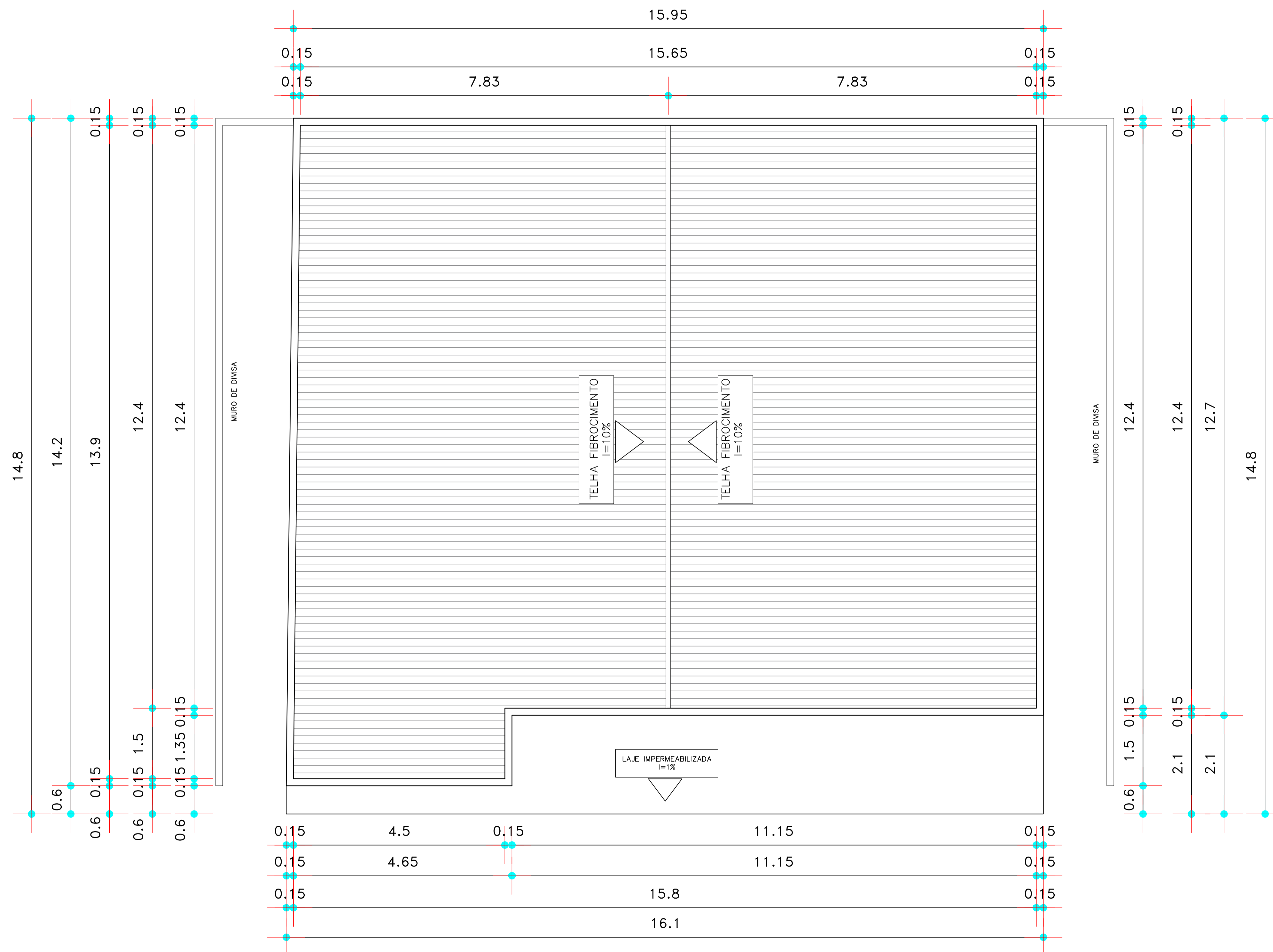
PLANTA BAIXA COBERTURA Esc: 1/50
