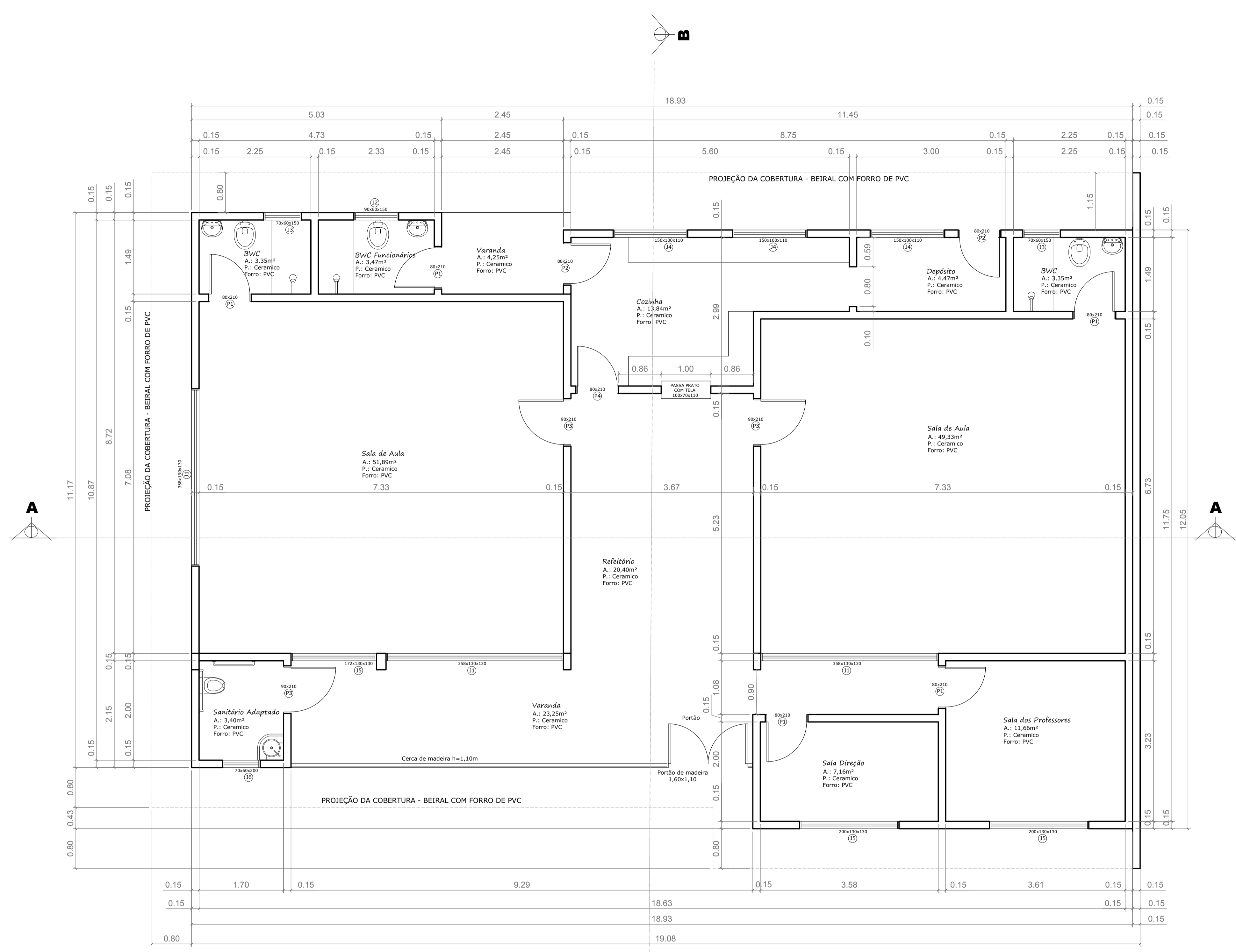
PLANTA BAIXA A. EXISTENTE: 64,65m 2 A. AMPLIAÇÃO: 152,30m 2 A. TOTAL: 216,95m 2 Esc.: 1/50
