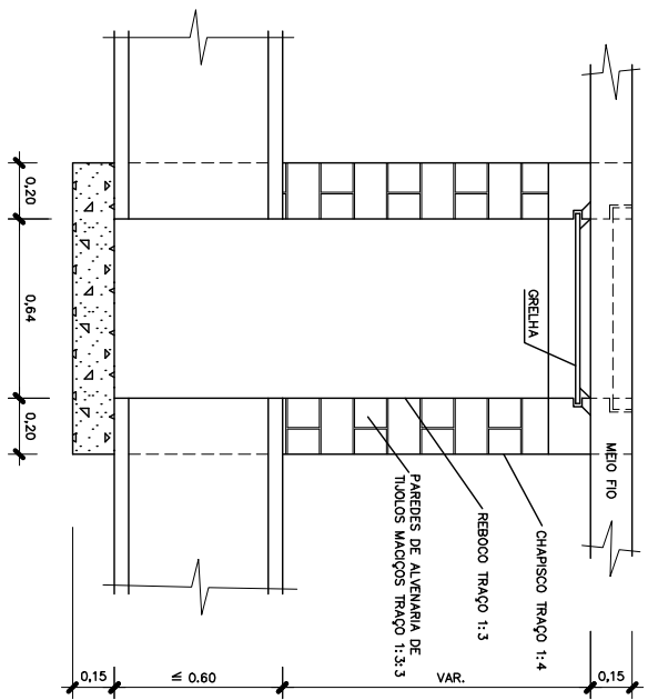
CORTE B-B
