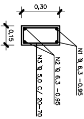
DETALHE DO MEIO FIO
