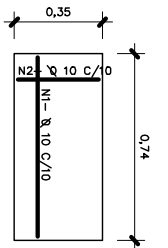
DETALHE DA TAMPA
