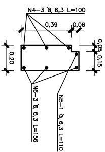
CORTE C-C
