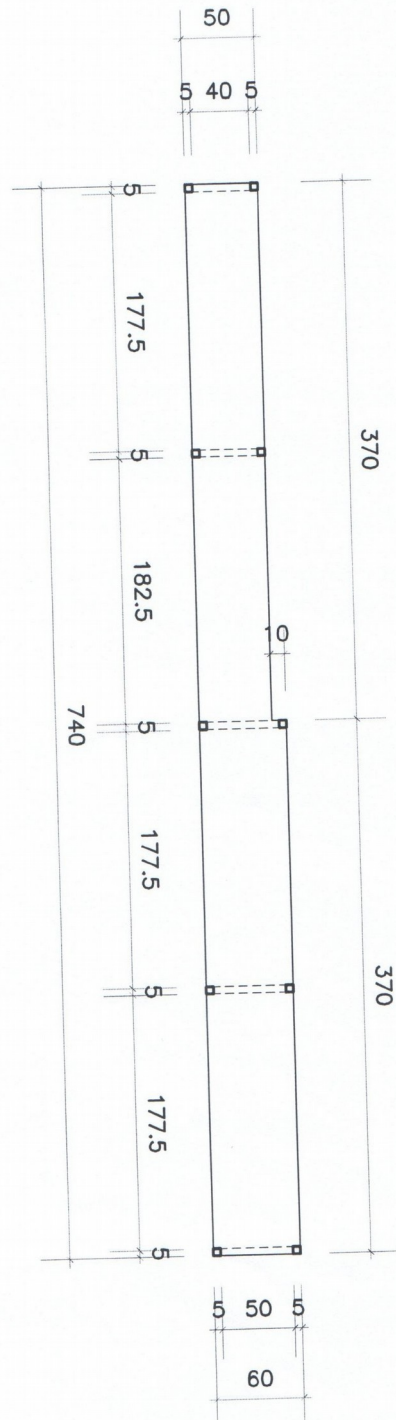
PLANTA BAIXA ESCALA: 1:50
