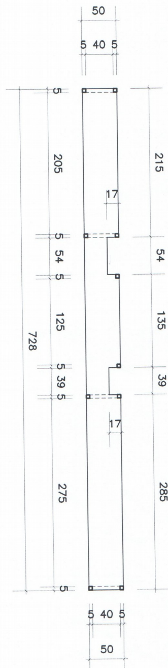
PLANTA BAIXA ESCALA: 1:50
