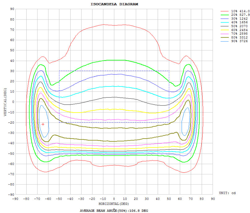
Figura 3 - Curva de distribuição de intensidade (isocandela)
