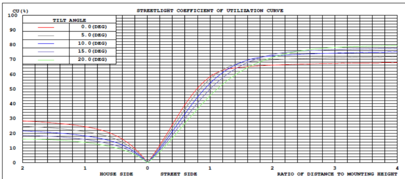
Figura 4 - Curva de coeficiente de utilização
