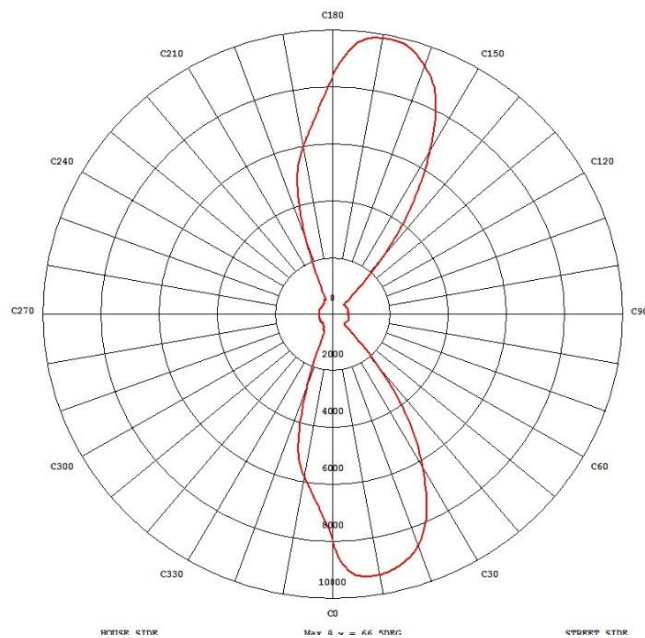
Figura 2 - Curva de distribuição de intensidade luminosa máxima
