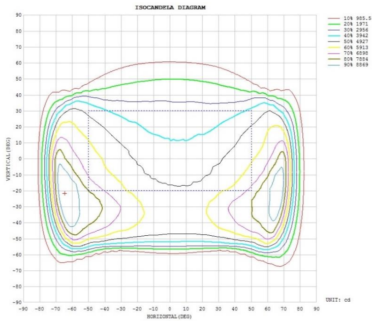
Figura 3 - Curva de distribuição de intensidade (isocandela)
