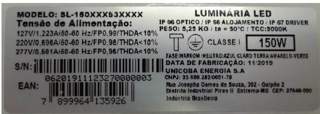
Foto 3 - Placa de identificação da amostra.
