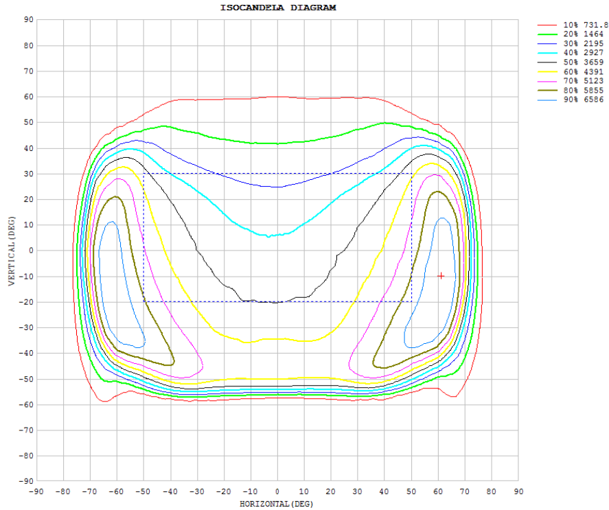
Figura 3 - Curva de distribuição de intensidade (isocandela)
