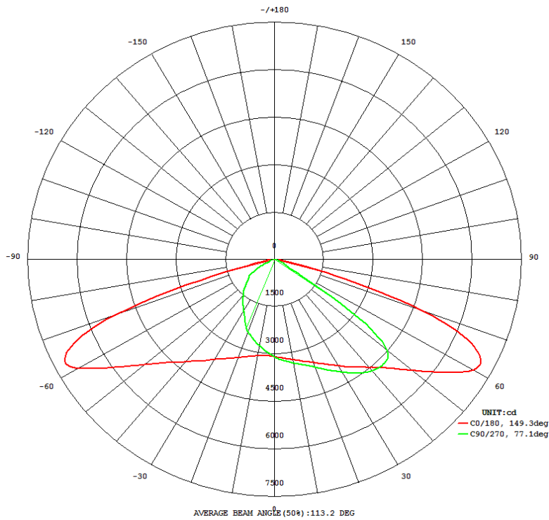
Figura 1 - Curva de distribuição de intensidade luminosa
