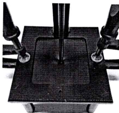
Figura 6. Ensaio de Resistência à Perfuração Estática.
